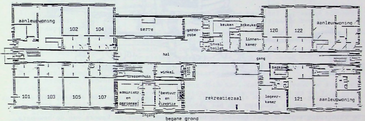
begane grond
