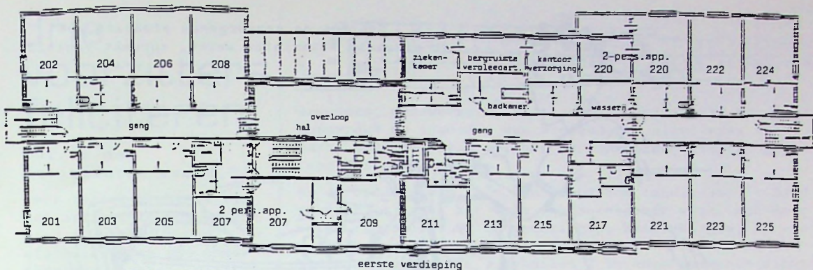
eerste verdieping
